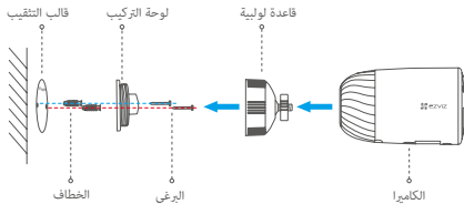
الشكل 2 التركيب باستخدام القاعدة اللولبية
